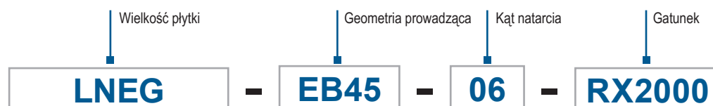
Płytki LNEG dla głowic Xfix HF86 i HF86B
