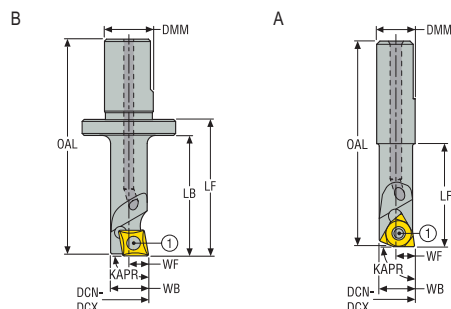
1 = Śruba mocująca płytkę
