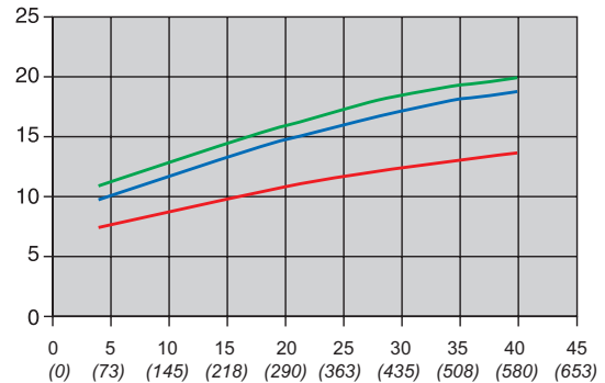
Przepływ chłodziwa przy różnych ciśnieniach
