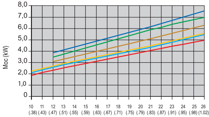
Średnica wiertła mm / (cale)
