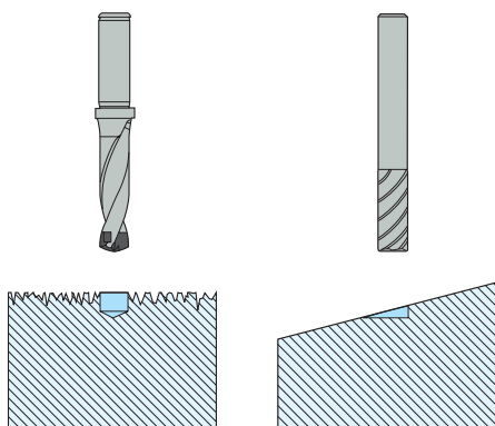
Kątowe wej. w materiał
