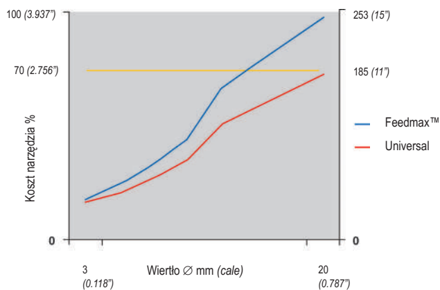
MRR, Szybkość usuwania materiału (cm 3 / min)
